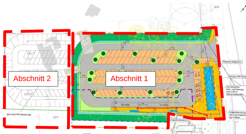
Abb. 7 Realisierung in zwei Etappen – Abschnitt 1 und 2 (Grundlage: Stationova Nov. 2021)
